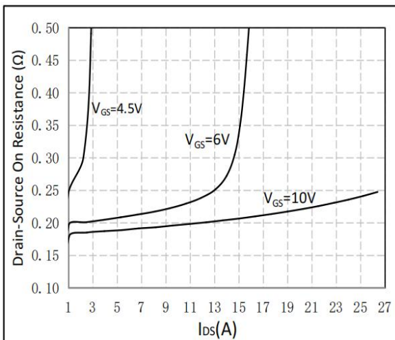
Fig3. R_{DS(on)} vs I_{DS}
