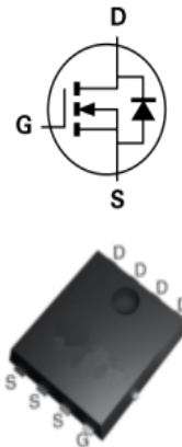
PDFN5x6
